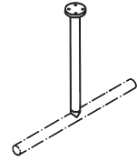
Support plafond Plafondsteun 33.7100B 250-3999 | ø 33
