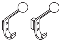
Porte-manteau et porte-chapeau Hoed- en jashaak 477.90.080 477.90.081 22 | 174 | 117 22 | 174 | 132
