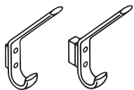
Porte-manteau et porte-chapeau Hoed- en jashaak 477.90.070 477.90.071 22 | 165 | 110 22 | 165 | 125
